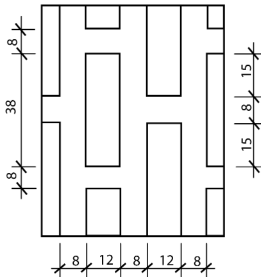
Рис. 1. Схема трафарету для влаштування контактної шару
