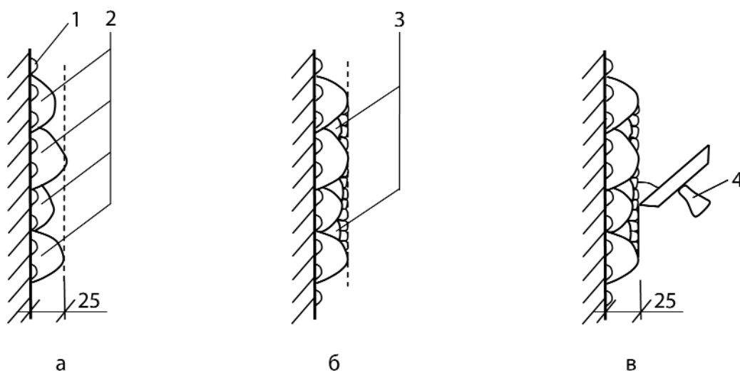
Рис. 2. Влаштування соленакопичувального шару легким багаторазовим накиданням: а — розчинна суміш, нанесена легким накиданням; б — додаткове накидання мікродозами розчинної суміші; в — легке розрівнювання з загладжуванням без ущільнення; 1 — контактний шар; 2 — розчинна суміш, накидана малими порціями; 3 — розчинна суміш, додатково накидана мікродозами; 4 — полутер.
